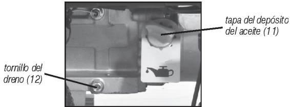
Fig. 21 – cambio de aceite
