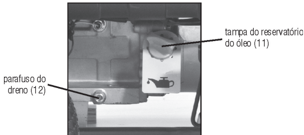
Fig. 21 – troca de óleo
