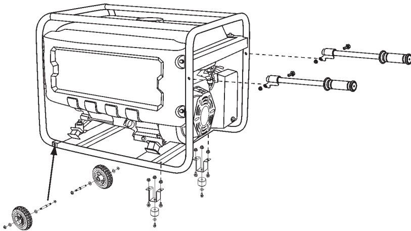
Fig. 6 – montagem dos pés, rodas e punhos
