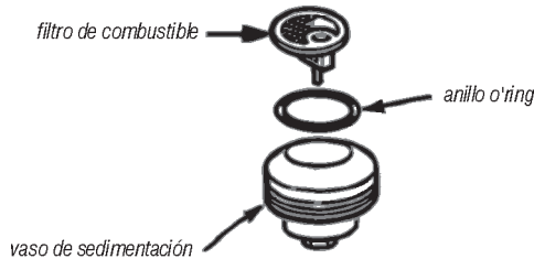
Fig. 25 – limpieza de los componentes
