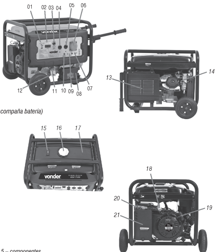
Fig. 5 – componentes
