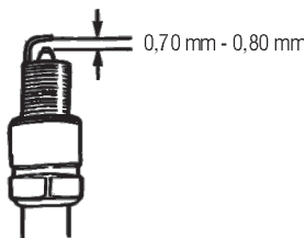
Fig. 27 – folga da vela
