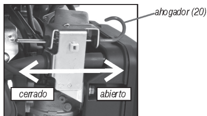
Fig. 13 – ahogador
