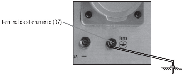
Fig. 15 – aterramento do gerador
