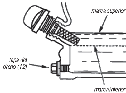
Fig. 8 – nivel de aceite
