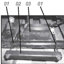
Fig. 20 – instalación de la batería
