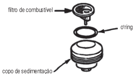
Fig. 25 – limpeza dos componentes
