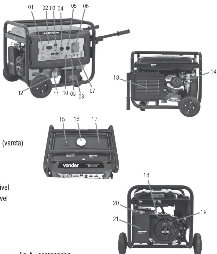
Fig. 5 – componentes
