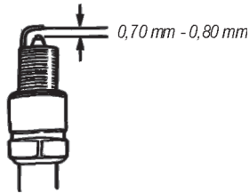
Fig. 27 – distancia de la bujía
