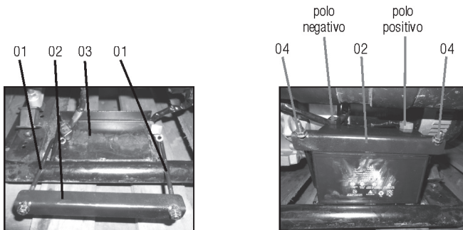
Fig. 20 – instalação da bateria
