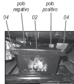
Fig. 20 – instalación de la batería
