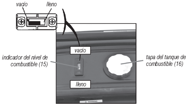
Fig. 9 – indicador del nivel de combustible
