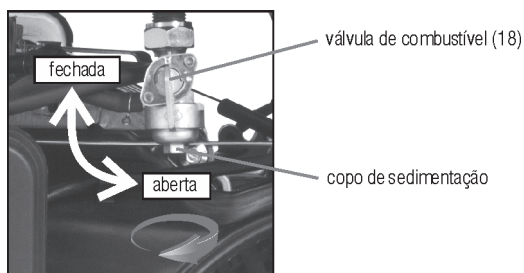
Fig. 24 – removendo copo de sedimentação
